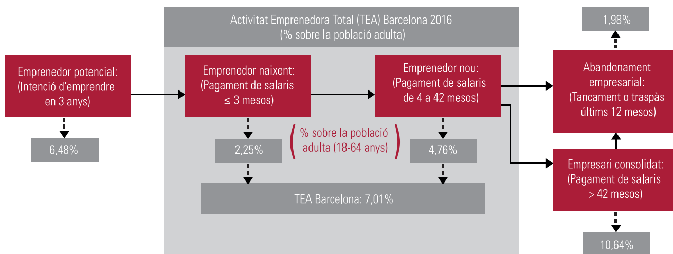
Gràfic 8. El procés emprenedor als països d'Europa basats en la innovació, 2016
