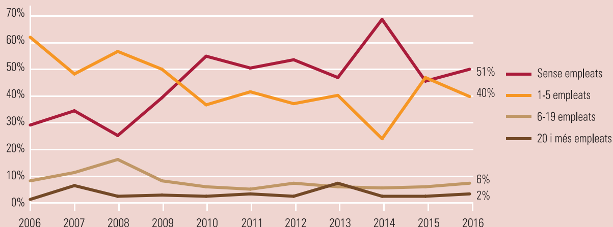
Gràfic 22. Evolució dels emprenedors en fase inicial (TEA) a Catalunya segons el volum en llocs de treball dels seus projectes de negoci en el període 2006-2016
