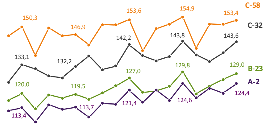
Intensitat mitjana diària a les vies d'alta capacitat d'accés a l'àrea metropolitana de Barcelona; 2015-2019
