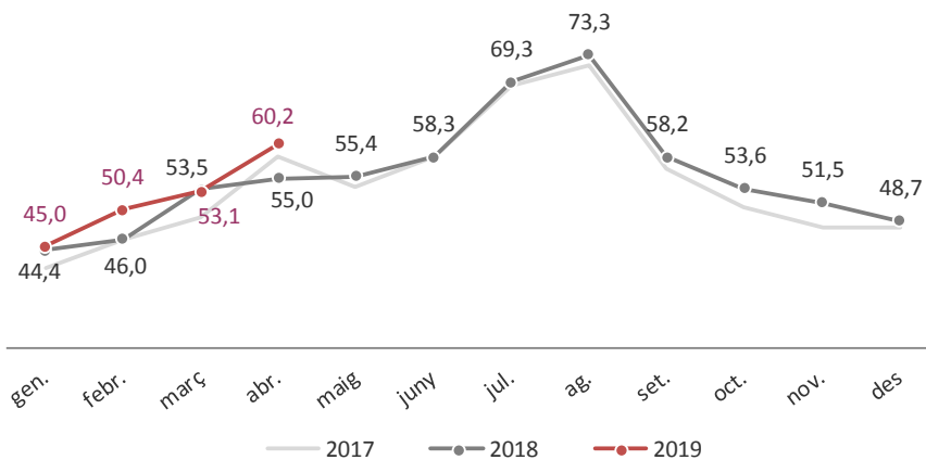
IMD (milers) Barcelona-Tarragona AP-7
